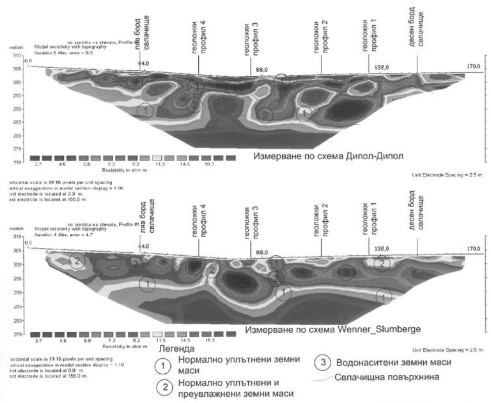
Фиг. 2 - геофизичен профил по оста на стената
